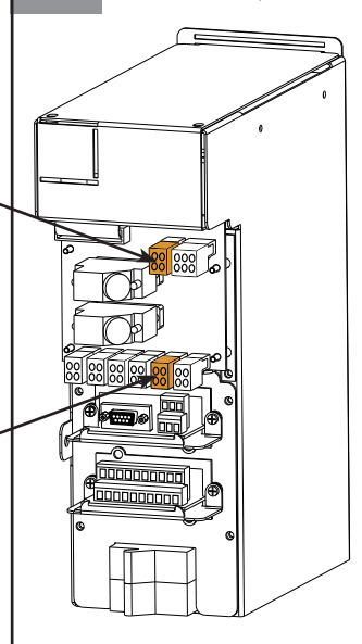
5.14-2 Interface QB612 :
