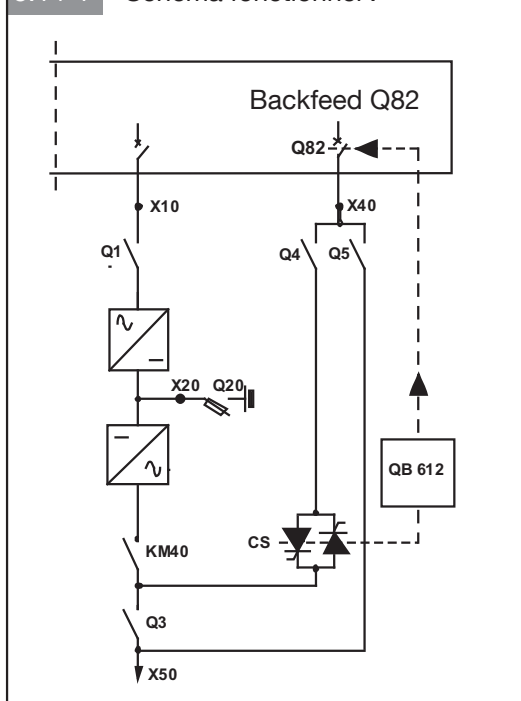
5.14-1 Schéma fonctionnel :
