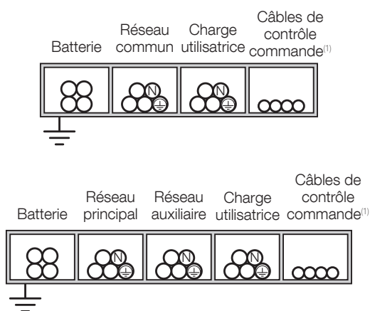
Installation correcte
